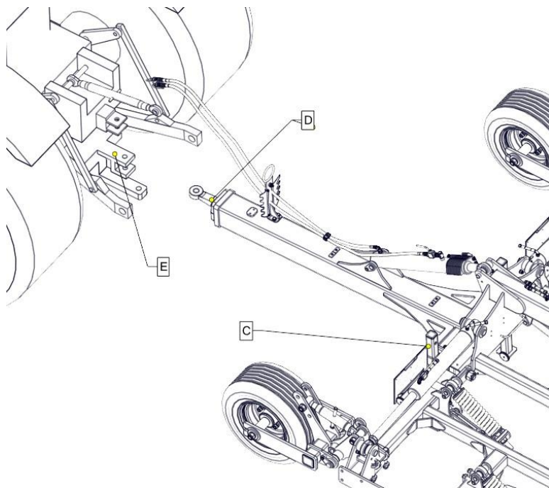
Рисунок 6: Подвешивание прицепного агрегата со сцепкой типа hitch
