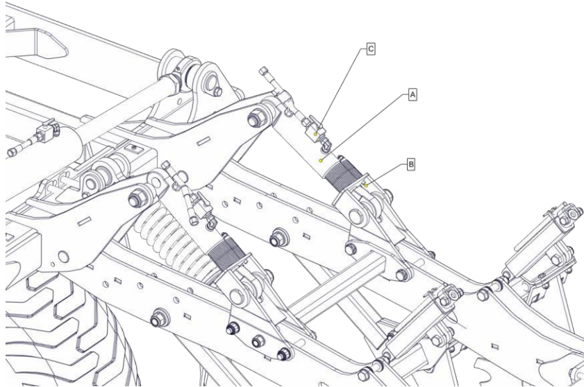
Рисунок 8: Регулирование рабочей глубины:
