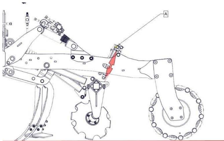
Рисунок 10: Регулирование бороны А
