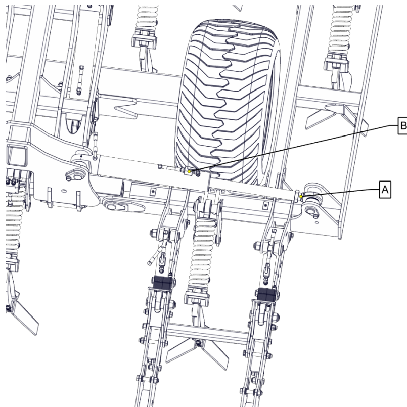
Рисунок 13: Регулирование гидравлики складывания
