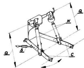
Рисунок 3: Подвеска тягача
