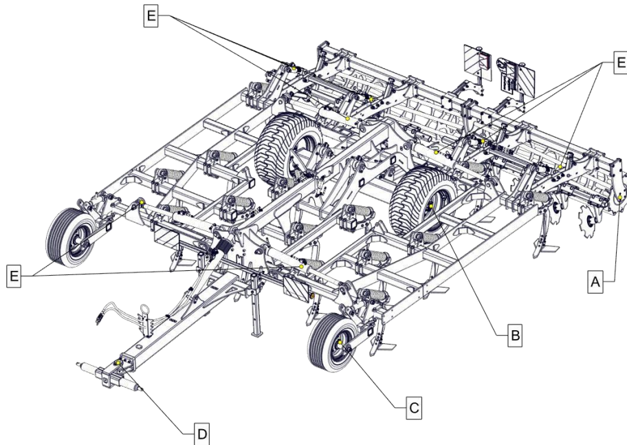
Рисунок:19 Смазочные точки CROSS HP
