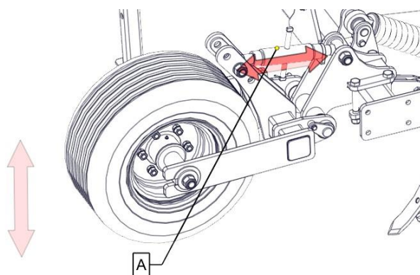
Рисунок:14 Регулирование глубины колеса
