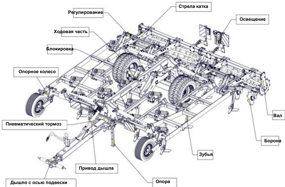
Рисунок 2: Конструкция ARES HP (5H; 6H, 8H)
