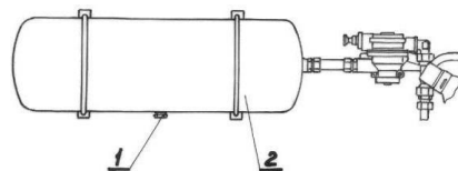
Рисунок 17: Слив воды из системы
