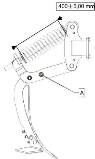
Рисунок 11: Защита зубца
