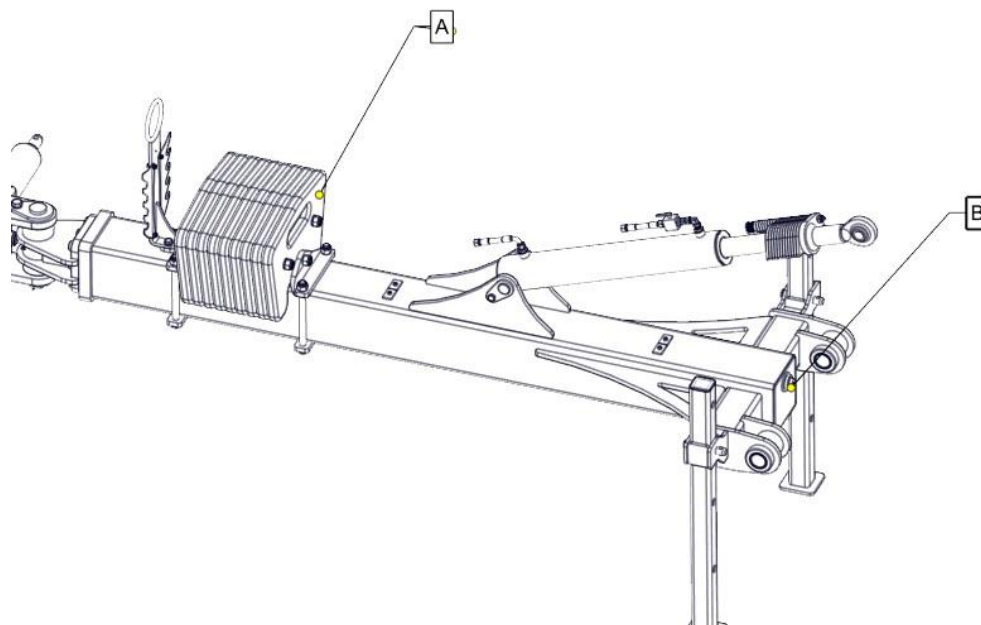
Рисунок: 18 Балласт
