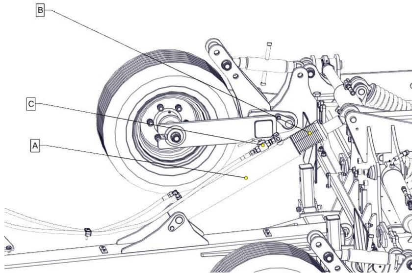
Рисунок 9: Регулирование привода на дышло
