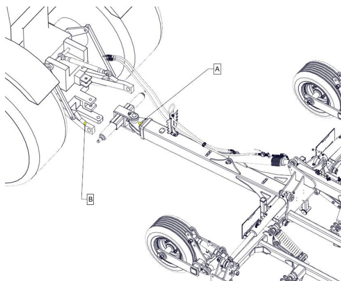
Рисунок 5: Подвешивание полунавесного агрегата
