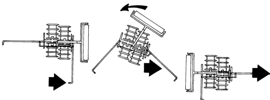
Рисунок:23 Каток-уплотнитель
